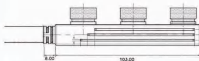
XYM15F-2P 1to3
