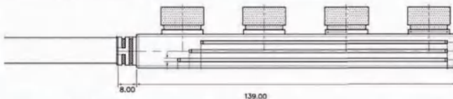
XYM15F-2P 1to4
