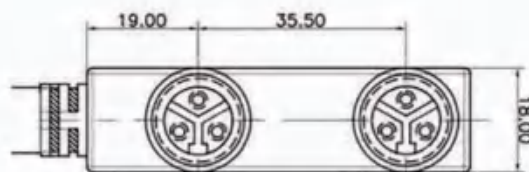
XYM15F-3P 1to2
