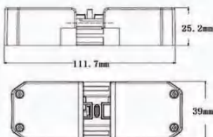
GST18-4P(DSC)
